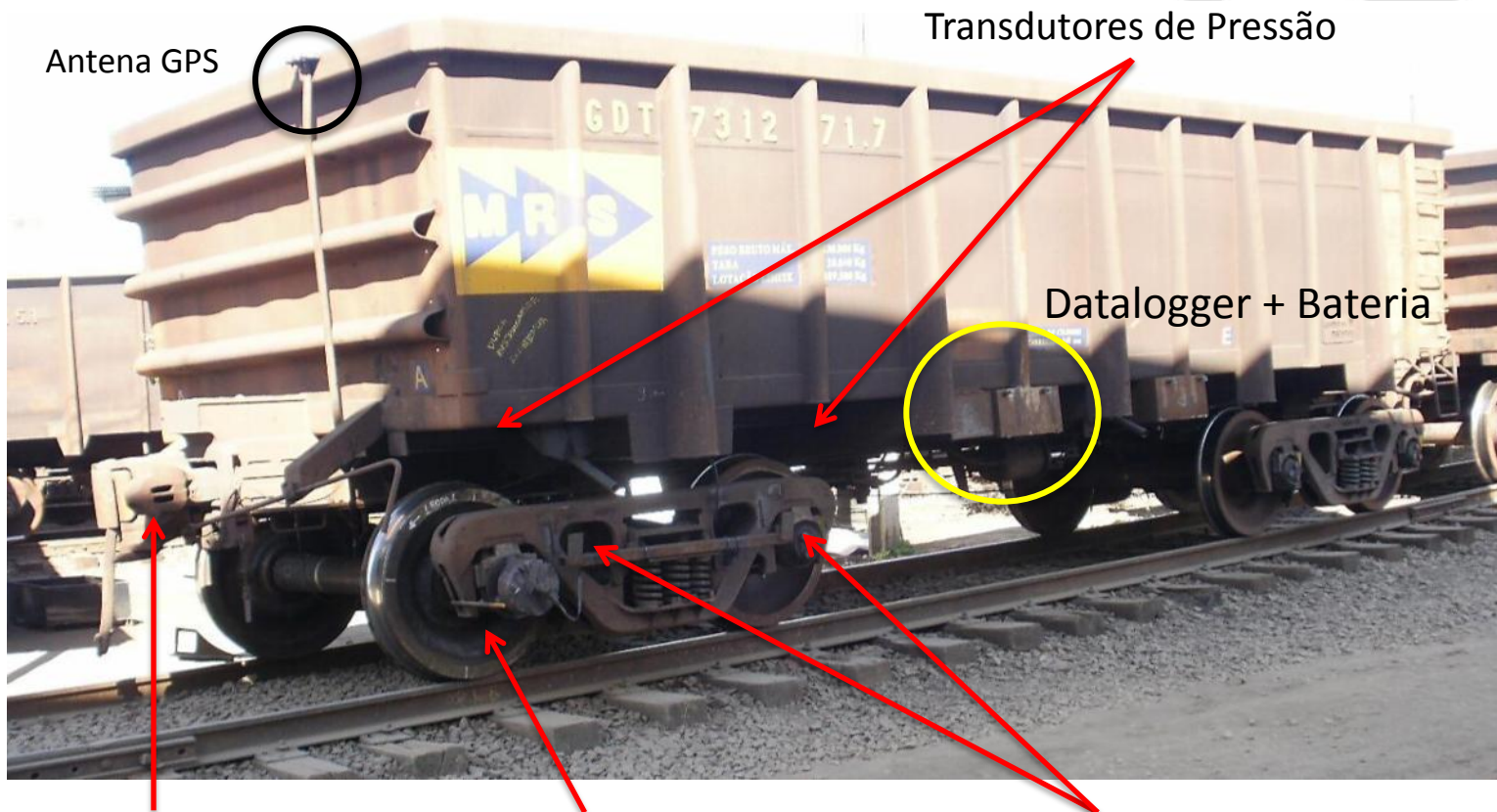
Engate Instrumentado
