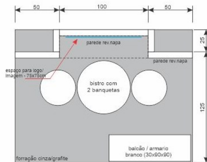
IMPLANTAÇÃO
